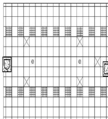
PLANTA FORRO LAUDOS ESCALA 1:100
