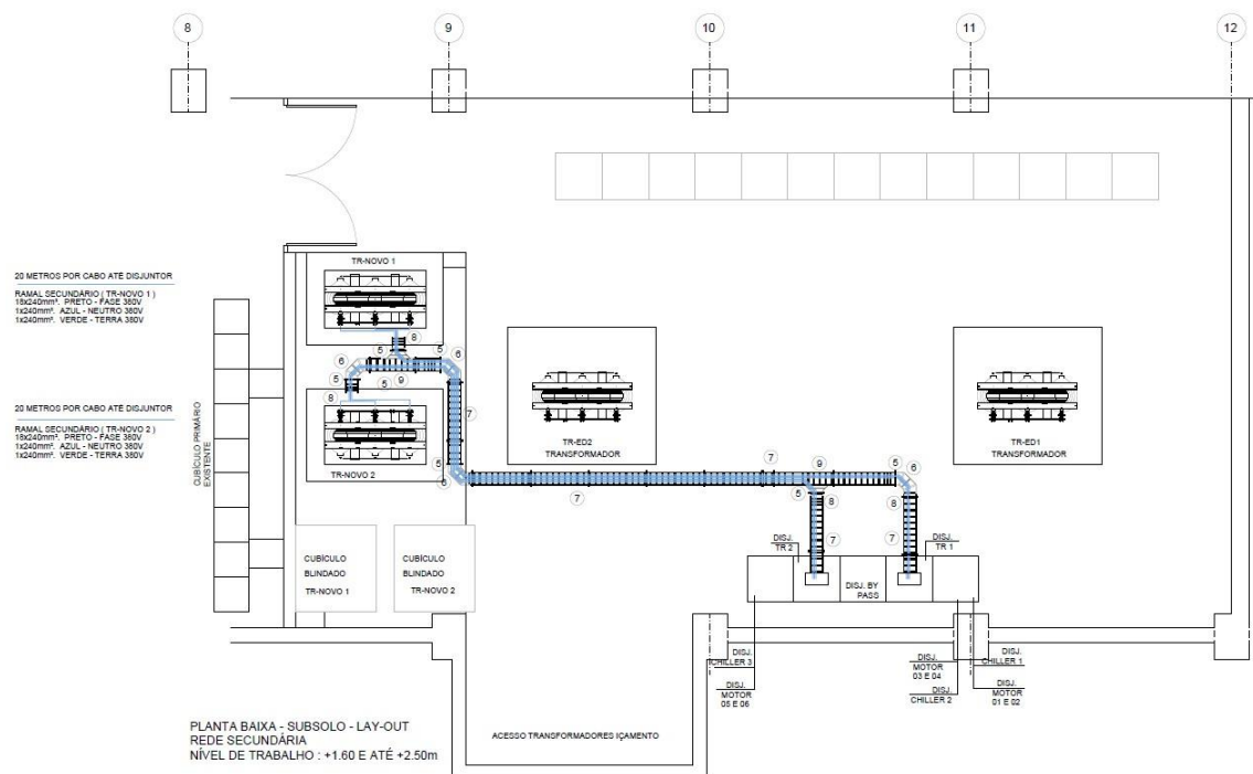
Figura 2 - Caminho do cubículo p/ os transformadores
